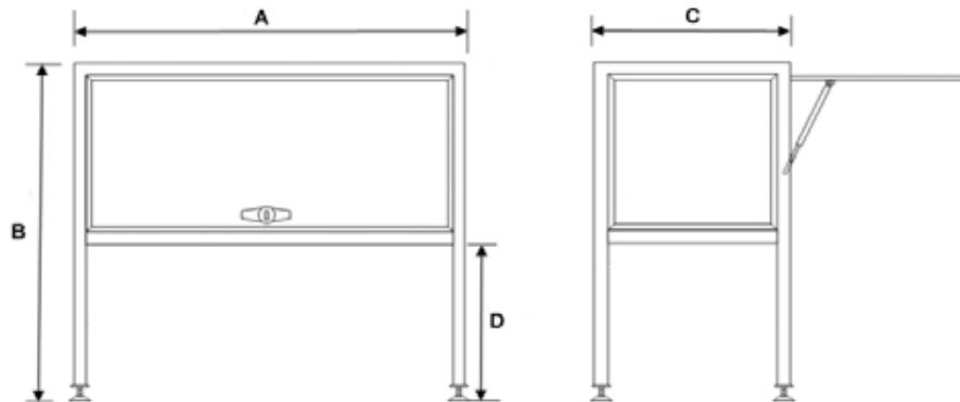
DIMENSIONS
